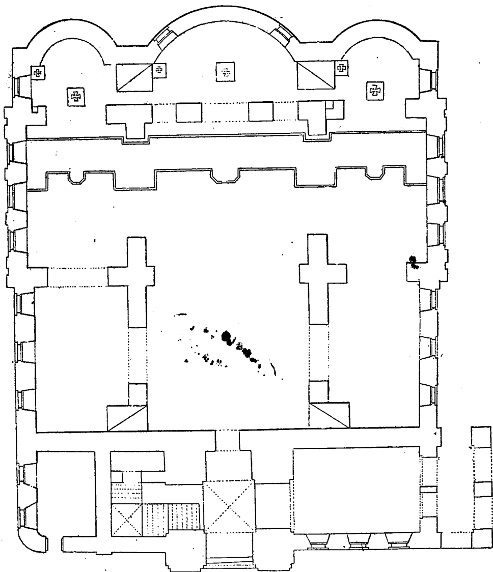
Планъ настоящей Георгіевской, что на Красной горѣ, церкви въ городѣ Москвѣ.
