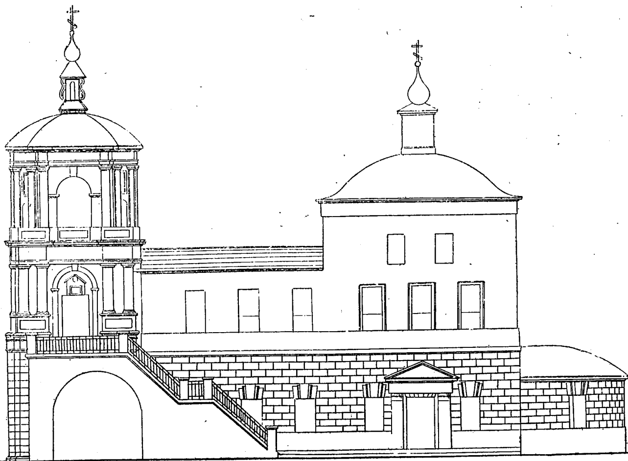
Фасадъ Московской Георгіевской, что на Красной горѣ, церкви до 1835 года.
