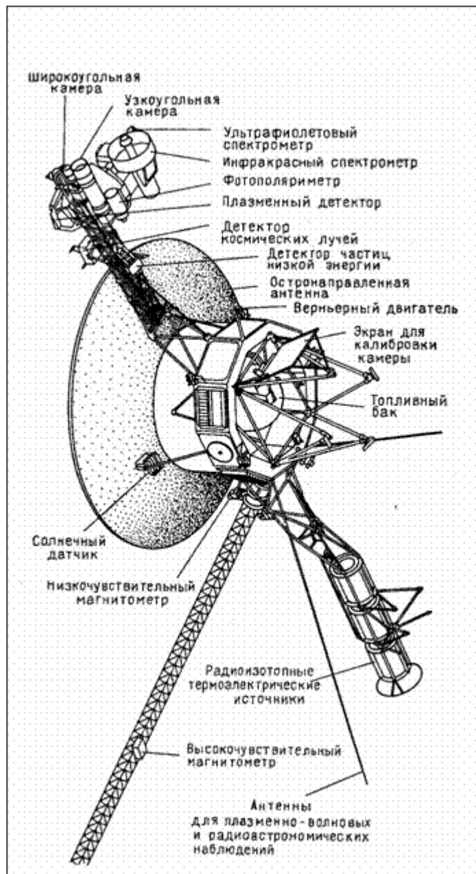
Рисунок 17 – Конструкция «Вояджеров»
