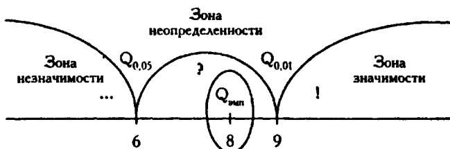
Рис. 1.7. Пример "оси значимости" для критерия Q Розенбаума
