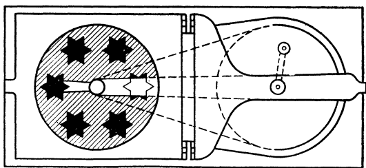
Рис. 180. Простейший проекционный хромаскоп.
