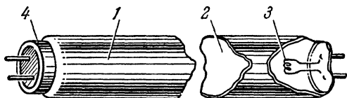
Рис. 204. Трубочатая люминесцентная лампа низкого давления.
