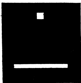
Рис. 126. При длительном рассматривании белого квадрата нижняя белая полоска исчезнет.
