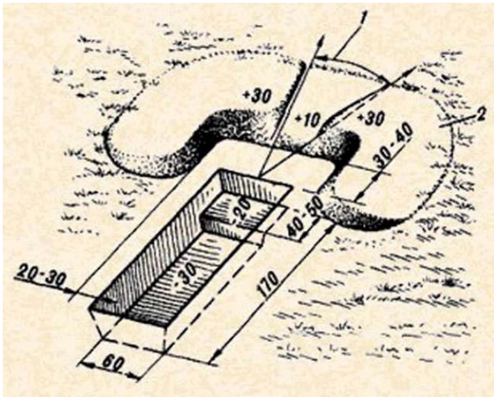
Рис. 21. Одиночный окоп для стрельбы из автомата лежа: 1 — сектор обстрела; 2 — бруствер
