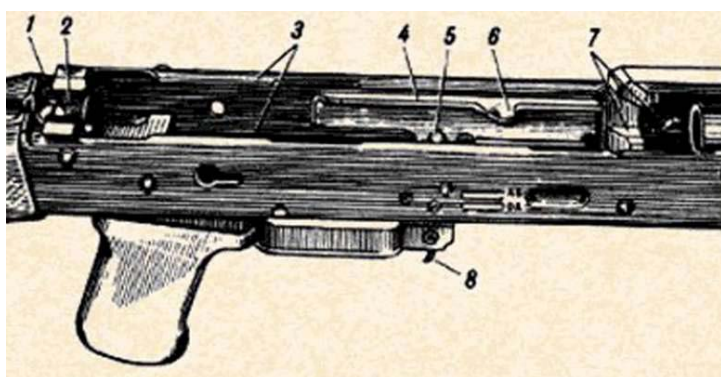
Рис. 28. Ствольная коробка:
