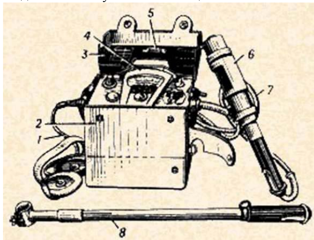
Рис. 121. Рентгенметр ДП-5А: 1 — кабель телефона; 2 — футляр; 3 — крышка футляра; 4 — измерительный пульт; 5 — контрольный препарат; 6 — зонд; 7 — кабель зонда; 8 — удлинительная штанга
